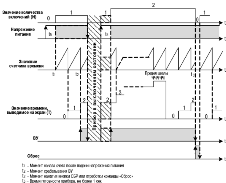
Рисунок 6.4 – Напряжение питания как сигнал управления счетом
