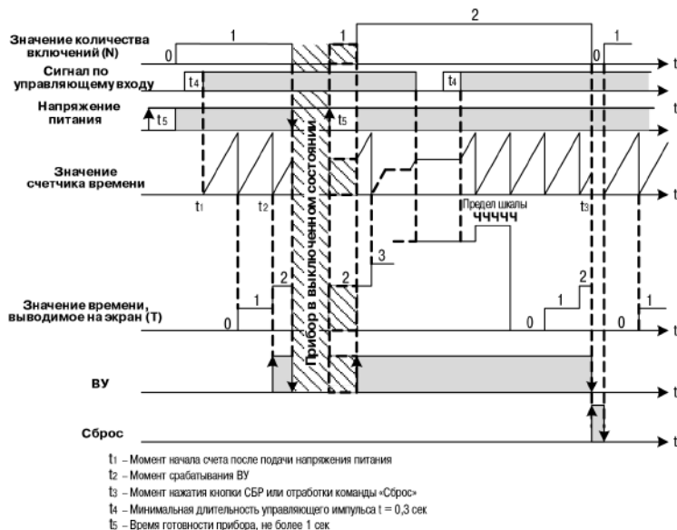
Рисунок 6.5 – Внешний сигнал управления счетом
